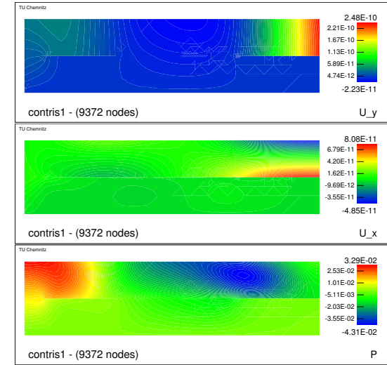
Abbildung 7: Verschiebungskomponenten und elektrisches Potential in Beispiel 1
