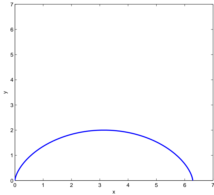
Ein Bogen der Zyckloide, a = 1
