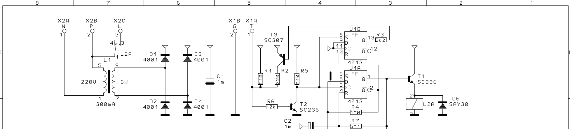
Licht-Zentralsteuerung mit LED-Tasten H. Haftmann, 20.02.00 HH_REL.SCH
